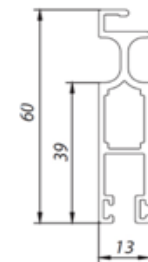
Rahmenprofil
