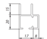
Laufschieneprofil Typ C Zargenprofil
